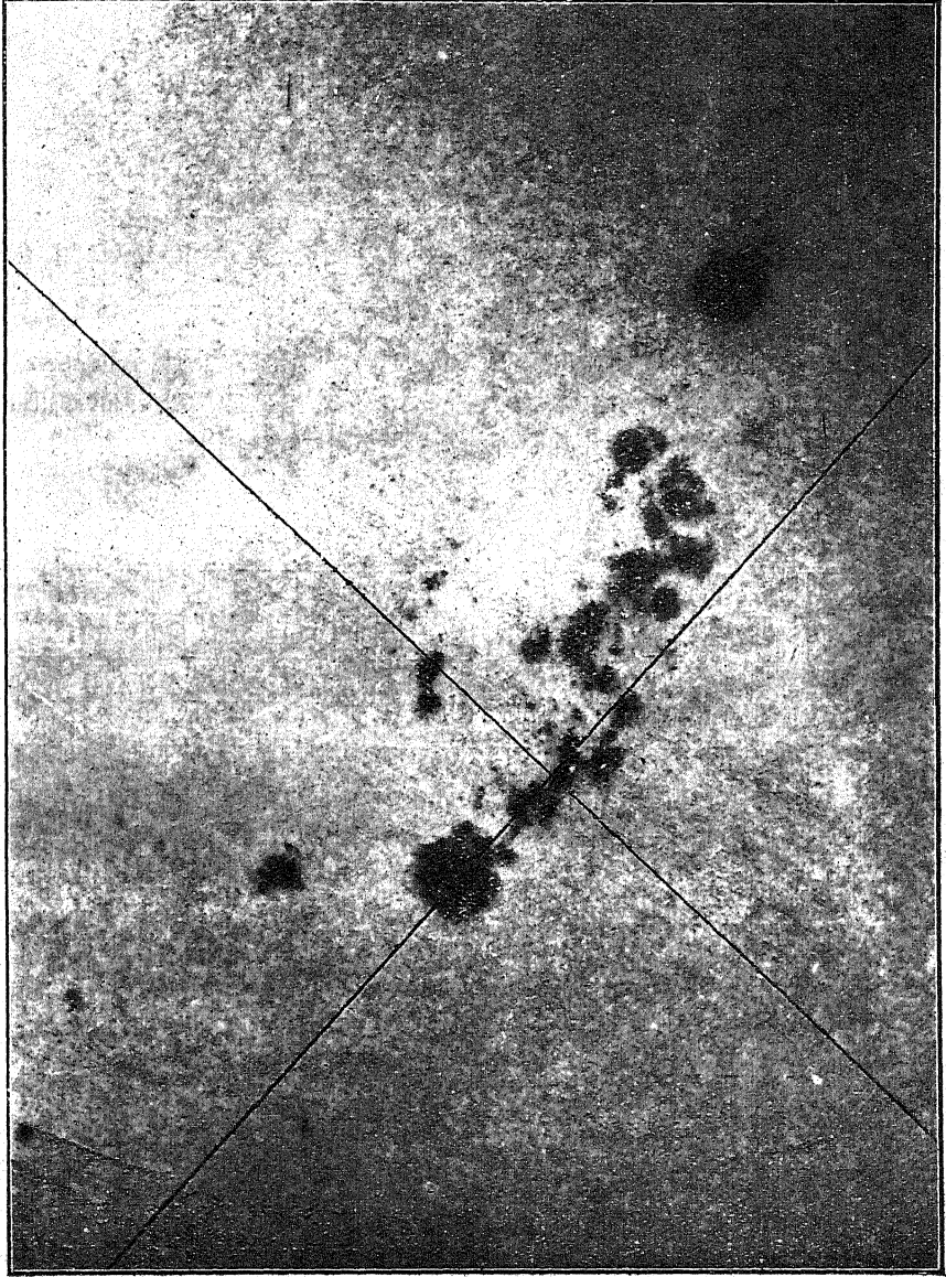
चित्र २१ — सूर्य के कलंक जो कभी-कभी बिना दूरबीन के भी देखे गये हैं । [ सौर-परिवार से ]
